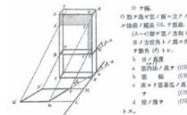
〈図版2〉 床上に於ける日射面の形状の作図法及び計算法(富永孟氏レポートより)
