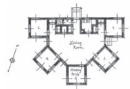
〈図版1〉 希望館平面図(富永孟氏レポートより)
