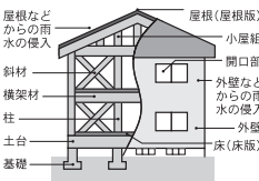
2階建ての場合の骨組み (小屋組、軸組、床組)等の構成
