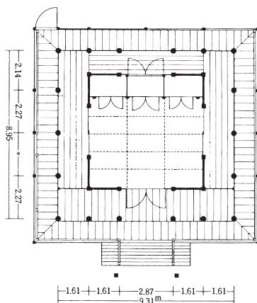
都久夫須麻神社本殿平面図
